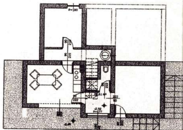
A középső, közösségi szint alaprajza
